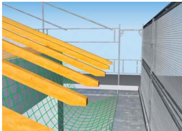
Figura 12 soluzione con rete di sicurezza montata presso lo sporto del tetto
