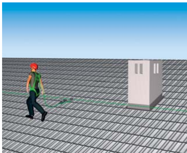
Figura 15 dispositivo anticaduta fisso (funi metallica)
