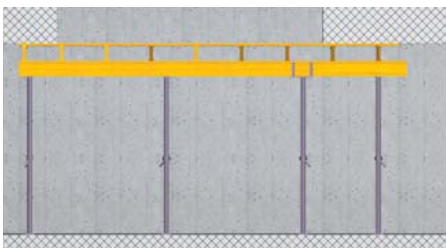
Figura 21 chiusura dell'apertura in una soletta con un ponteggio di ritenuta
