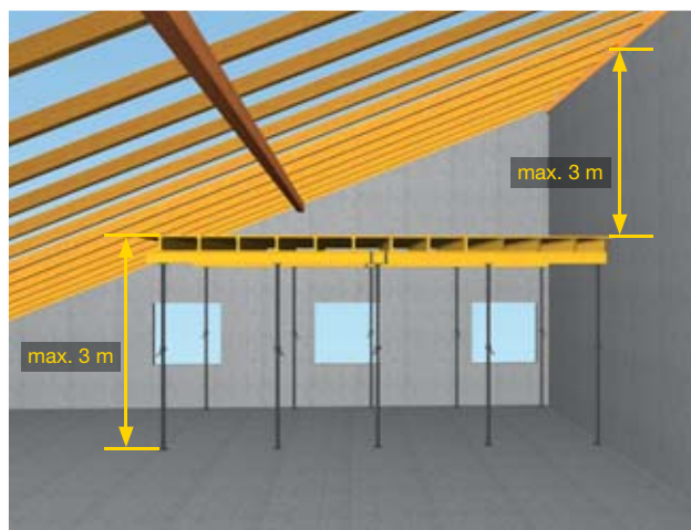
Figura 11 ponteggio di ritenuta montato al di sotto di una struttura portante
