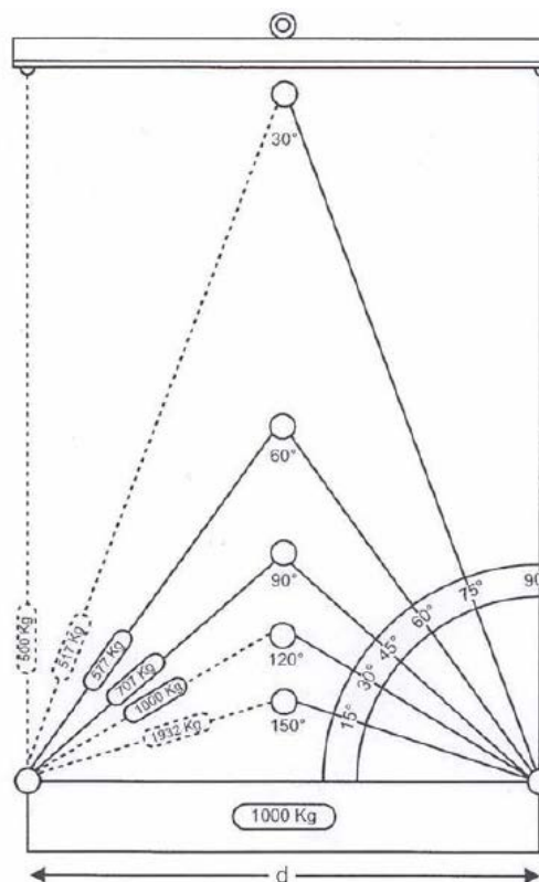
Variatione della forza sui bracci di un tirante per effetto dell'angolo \beta per un carico di 1000kg.
