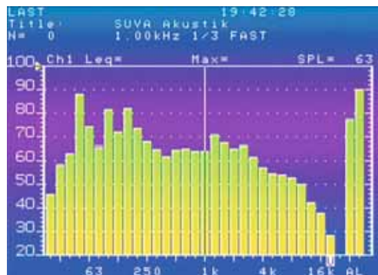
Figura 52: rappresentazione di uno spettro in banda d'ottava sullo schermo di un analizzatore di frequenza.
