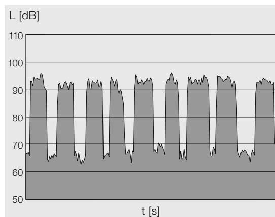
Figura 23: rumore intermittente (segnale di allarme).
