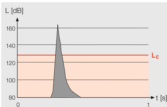
Figura 13: livello di esposizione sonora L_E .
