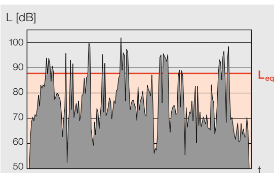
Figura 12: andamento temporale del livello di pressione sonora L(t) e del livello sonoro equivalente L_{eq} .
