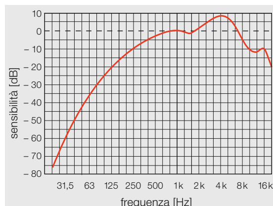
Figura 32: risposta in frequenza del campo sonoro libero attraverso l'orecchio esterno e medio fino all'orecchio interno.
