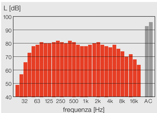
Figura 19: rumore a banda larga.
