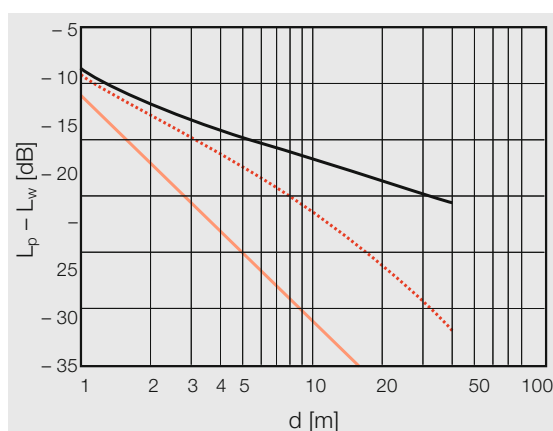
Figura 58: curva di propagazione del suono.
