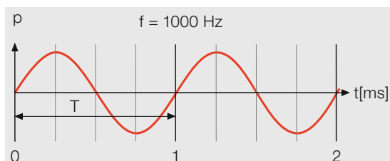
Figura 5: periodo e frequenza: oscillazione di periodo T = 1 \text{ ms} = 1000 oscillazioni al secondo = 1000 Hz.
