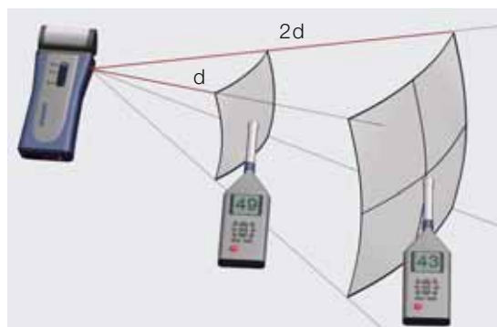
Figura 26: la pressione sonora si riduce con l'aumento della distanza dalla sorgente puntiforme.
