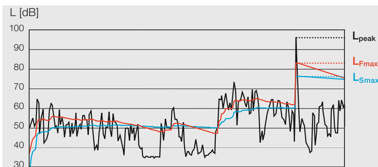
Figura 47: valore massimo «peak» e valori effettivi «fast» e «slow» di un segnale acustico.
