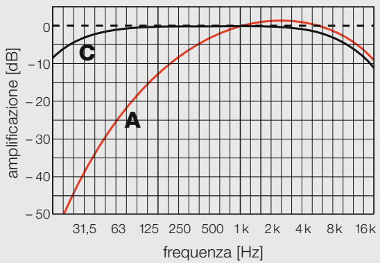
Figura 11: filtri di ponderazione A e C.
