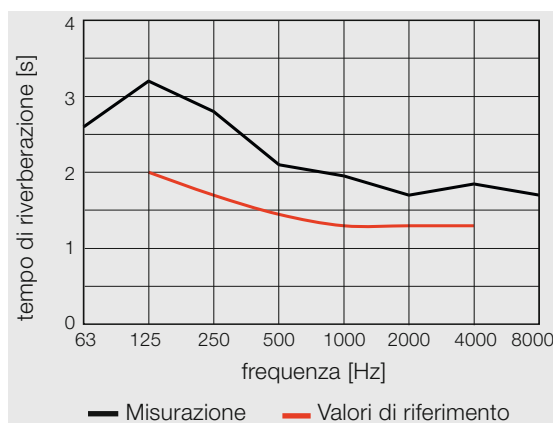
Figura 57: rappresentazione dei tempi di riverberazione.
