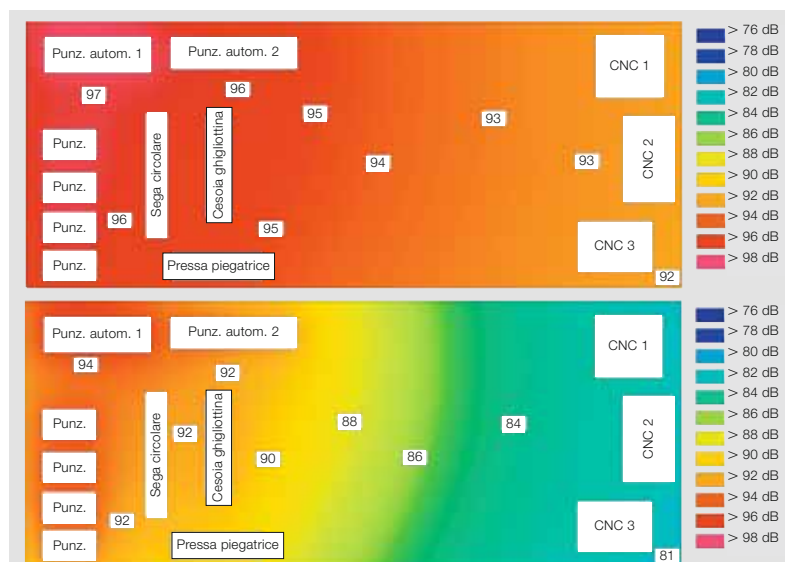
Figura 78: ripartizione dei livelli sonori in un locale di fabbricazione senza (in alto, DL_2 = 2,1 dB) e con soffitto fonoassorbente (in basso, DL_2 = 4,3 dB).
