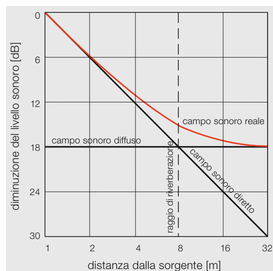
Figura 27: interferenza tra il campo sonoro diretto e il campo sonoro diffuso (raggio di riverberazione 8 m).
