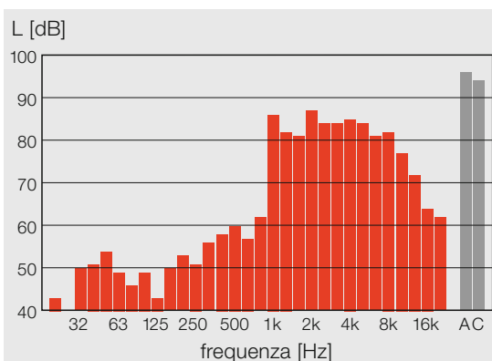
Figura 21: rumore ad alta frequenza.
