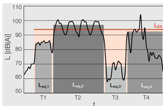
Figura 60: esposizioni al rumore variabili e livello di esposizione al rumore L_{EX} .
