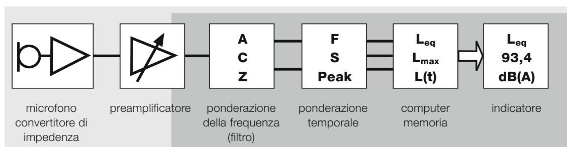
Figura 46: struttura semplificata di un fonometro integratore. I fonometri di nuova generazione sono spesso in grado di applicare simultaneamente diversi filtri di frequenza e diverse ponderazioni temporali. Oggi le funzioni a sfondo grigio sono solitamente realizzate con la tecnologia digitale.
