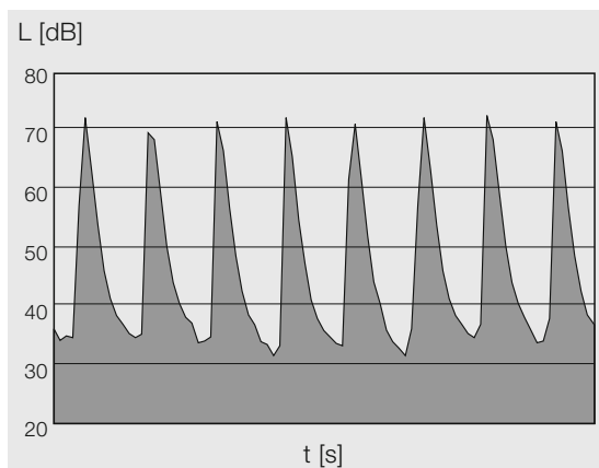
Figura 24: rumore impulsivo
