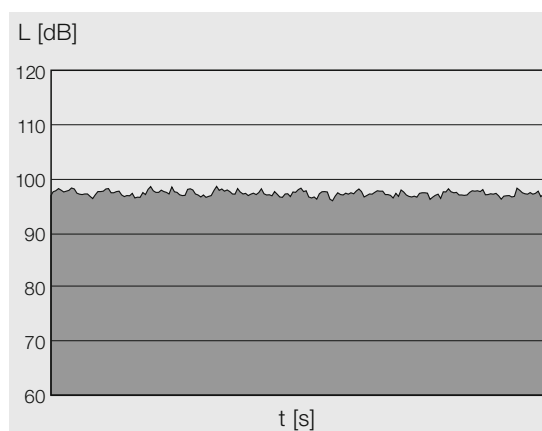
Figura 22: rumore continuo (sala di tessitura).
