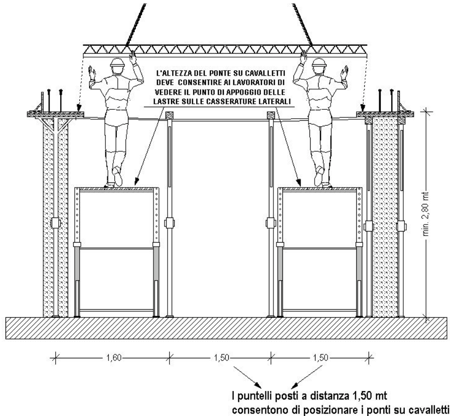
fig. 32 – posa lastre dal basso, operando su ponte su cavalletti
