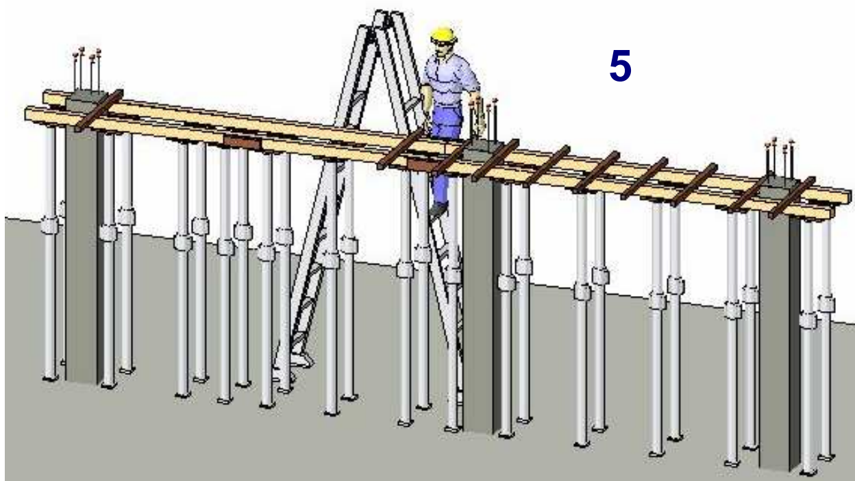
fig. 17 - posa in opera stecchetti trasversali ai correnti
