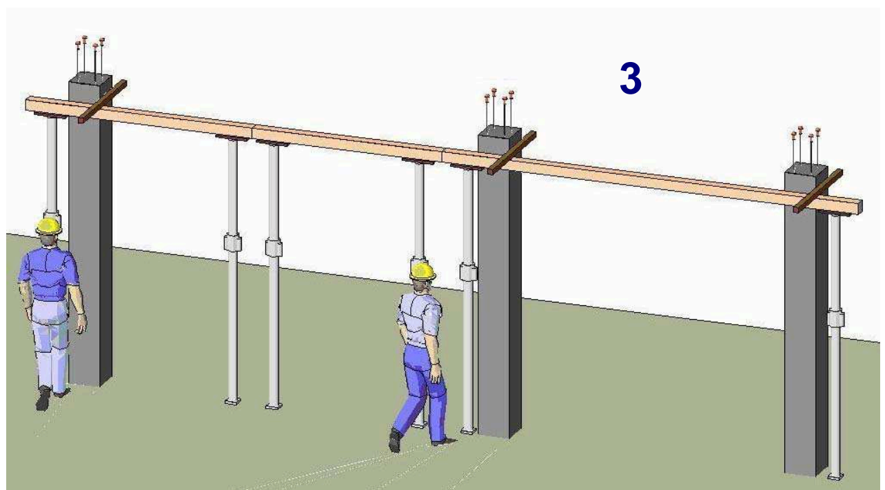
fig. 15 - posa in opera puntelli e travetto di sostegno banchinaggio
