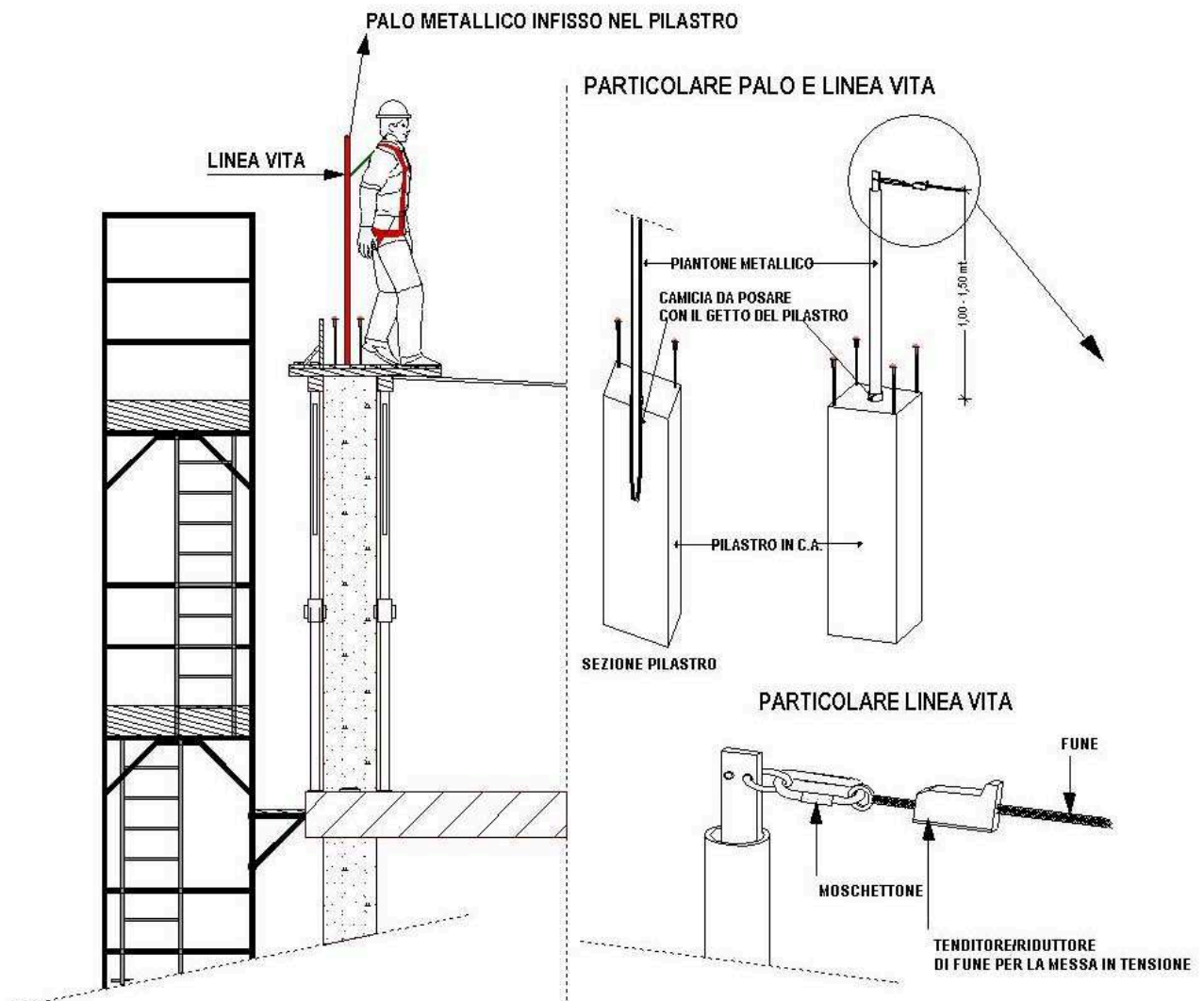
Fig. 32 – particolari linea vita
