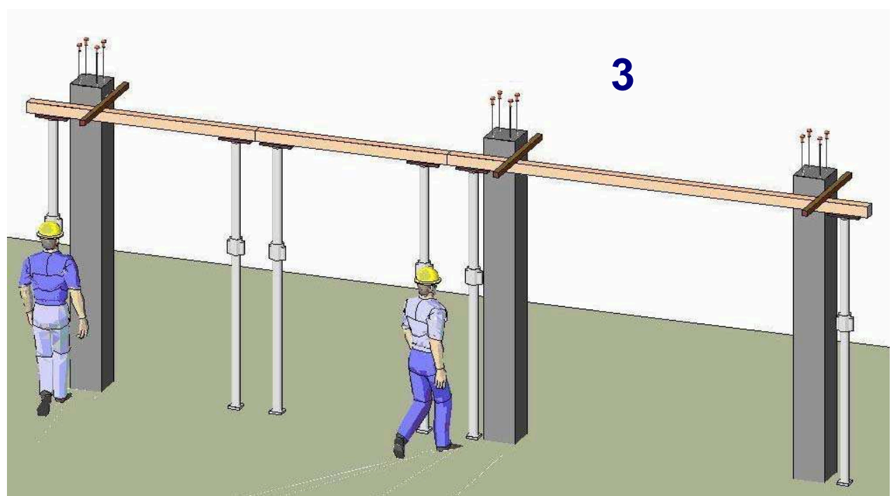
fig. 23 - posa in opera puntelli e travetto di sostegno banchinaggio
