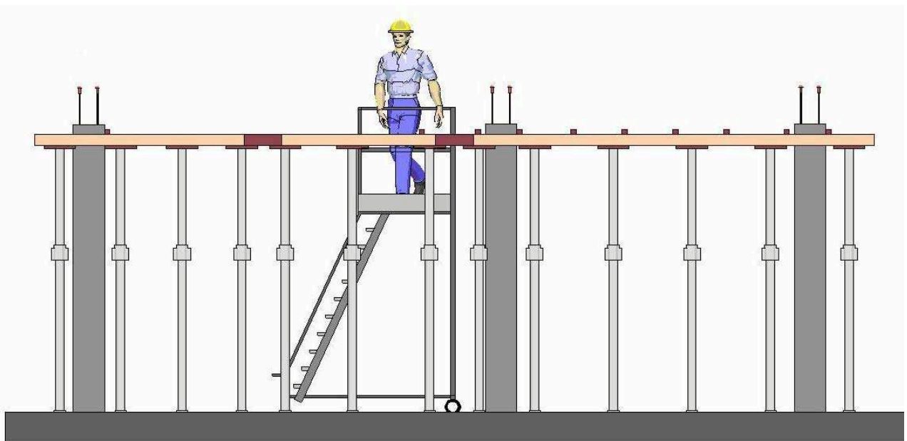
fig. 27 - posa in opera banchinaggio con uso scala a castello di dimensioni idonee alla lavorazione
