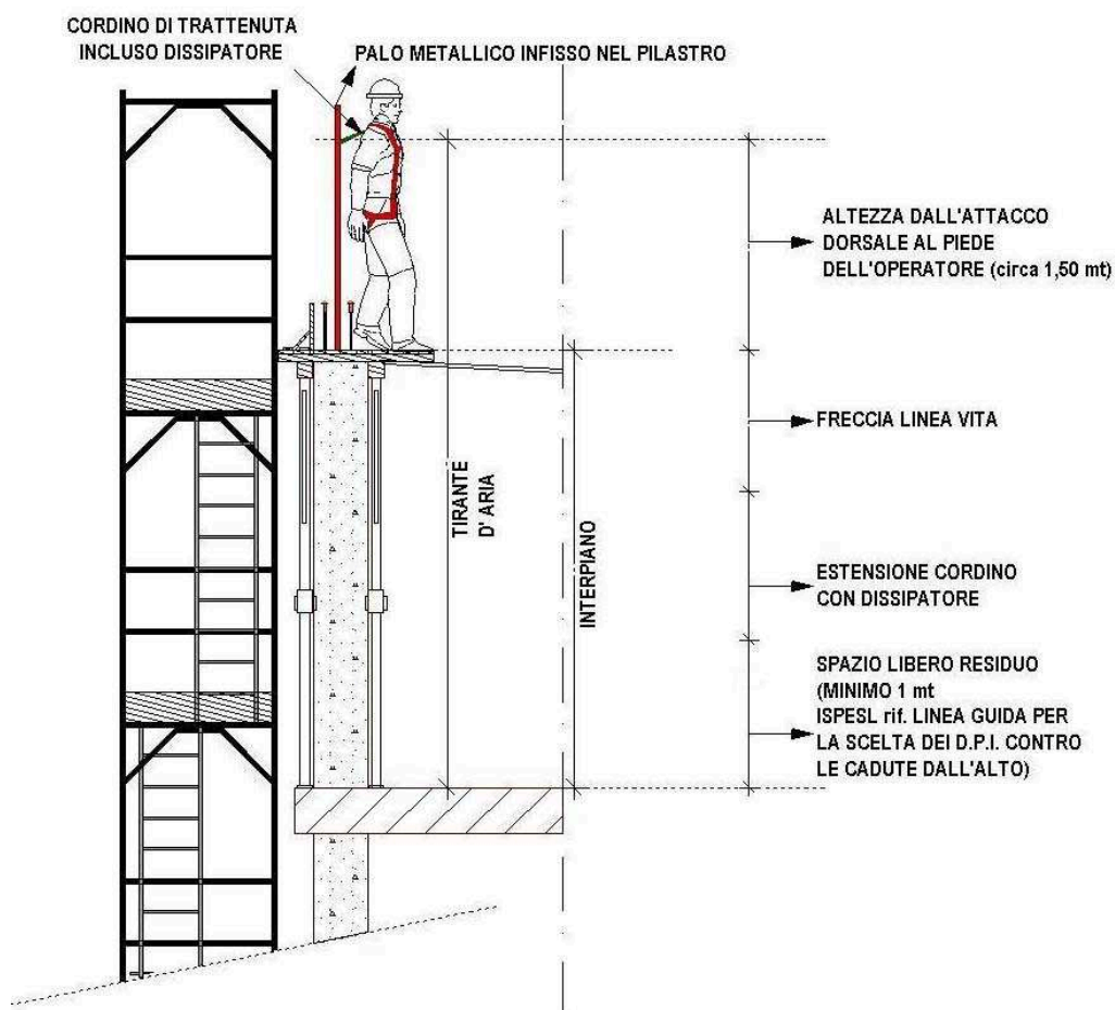
fig. 30 – Posa lastre con uso linea vita tesata tra i montanti annegati nel getto dei pilastri – verifica tirante d’aria
