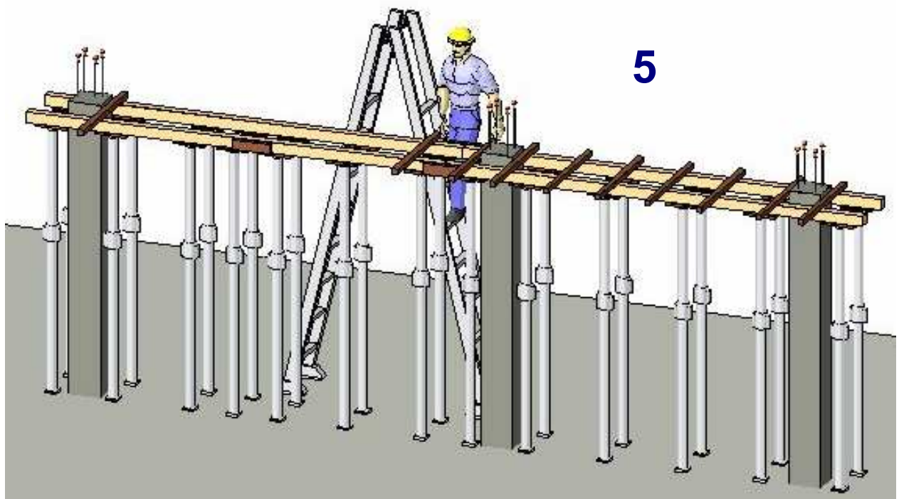
fig. 25 - posa in opera stocchetti trasversali ai correnti
