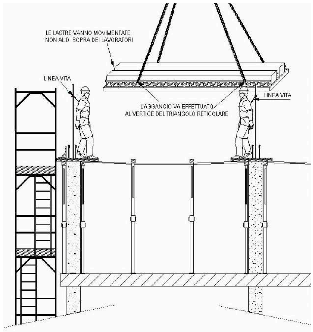
fig. 26 – Posa in opera lastre con ausilio linea vita tesata parallelamente al banchinaggio travi laterali
