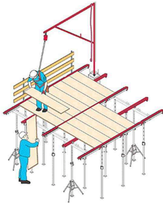
fig. 61 – Esempificazione sistema Alsina per posa dall'alto intavolato continuo
