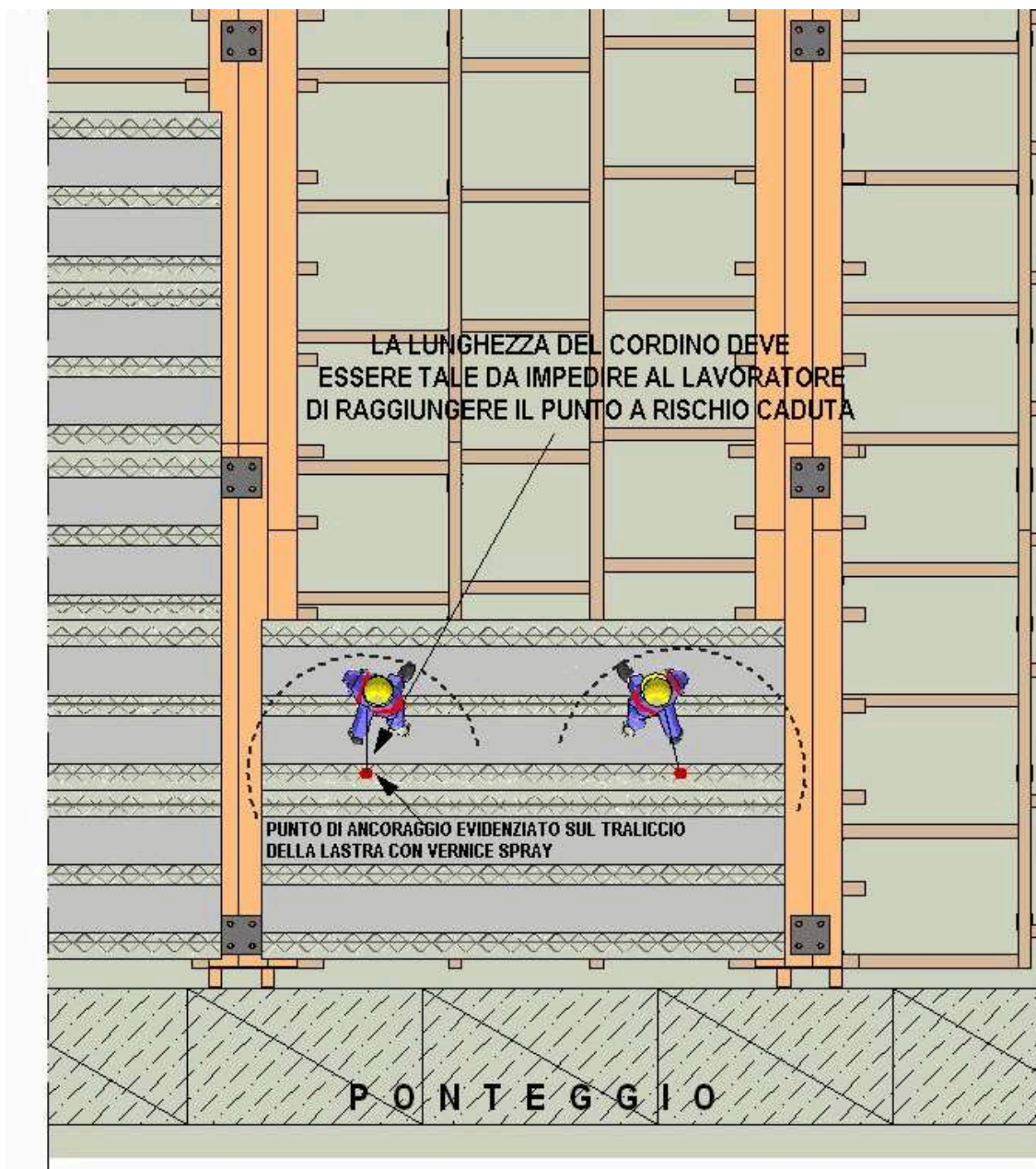
fig. 24 – Ancoraggio cordino in modo da garantire la completa trattenuta in ogni direzione
