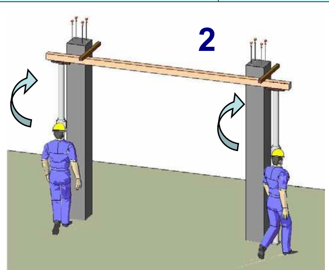
fig. 22 - innalzamento puntello e corrente a livello quotato per il banchinaggio
