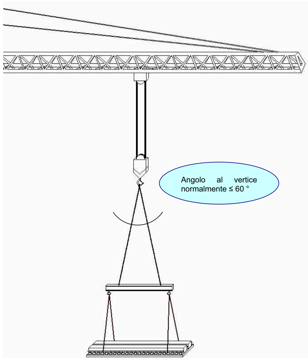
fig. 10 – Sollevamento carico con angolo al vertice inferiore ai 60° - uso di bilancini
