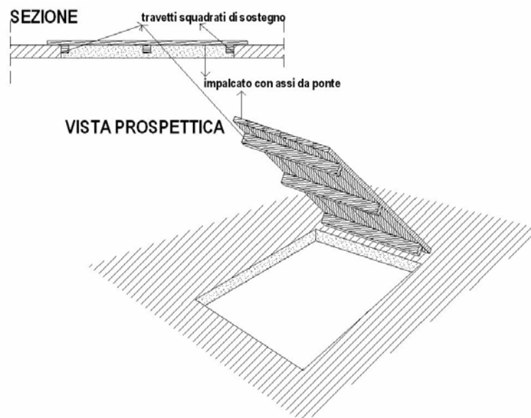
fig. 67 – Intavolato per chiusura buchi o forometri varie
