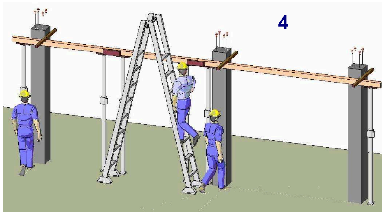
fig. 16 – collegamento - controvento correnti attigue con scala portatile
