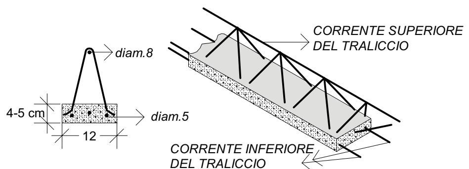
fig. 2 – travetti con base in c.a. normale
