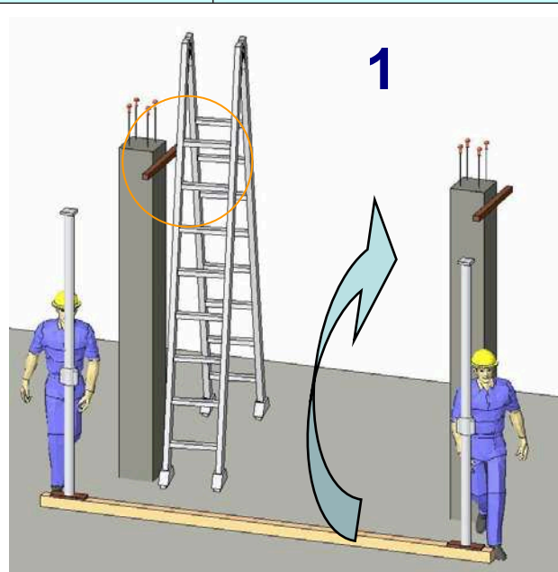
fig. 21 - posa in opera listelli di riferimento chiodati al pilastro e allestimento cavalle a terra con chiodatura puntelli al corrente di sostegno
