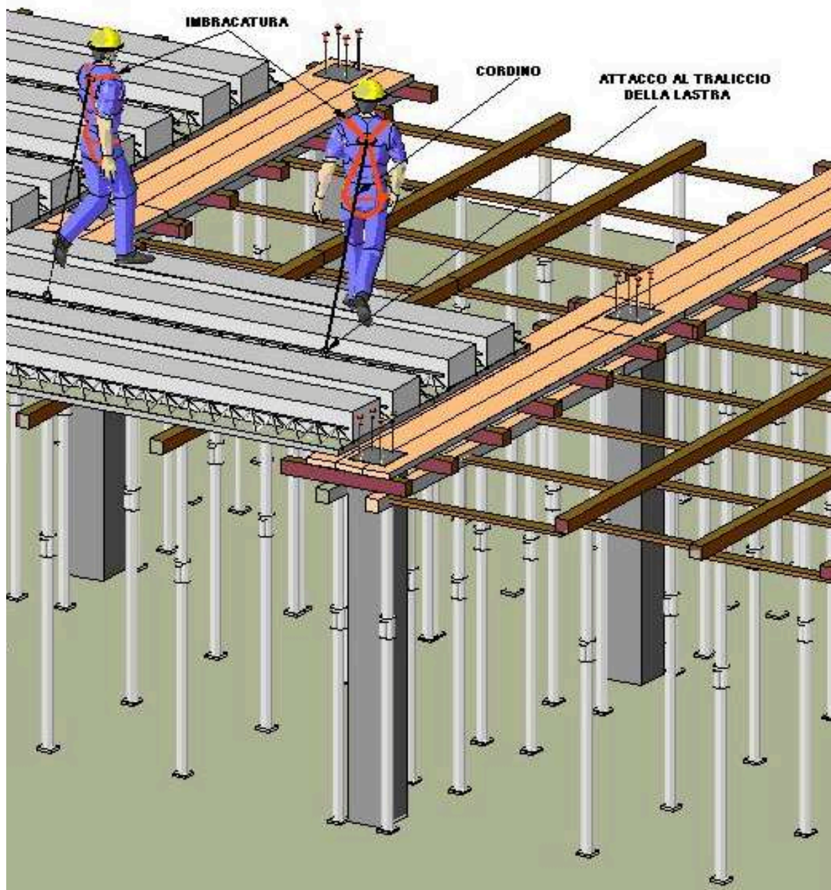
fig. 23 - posa lastre con lavoratori in quota ancorati al traliccio delle lastre già posate, con cordini di trattenuta senza dissipatore
