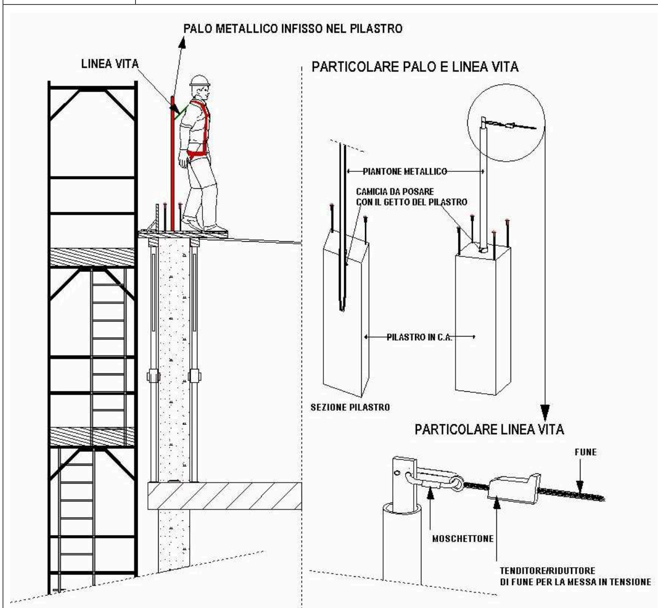
fig. 29 - particolari linea vita
