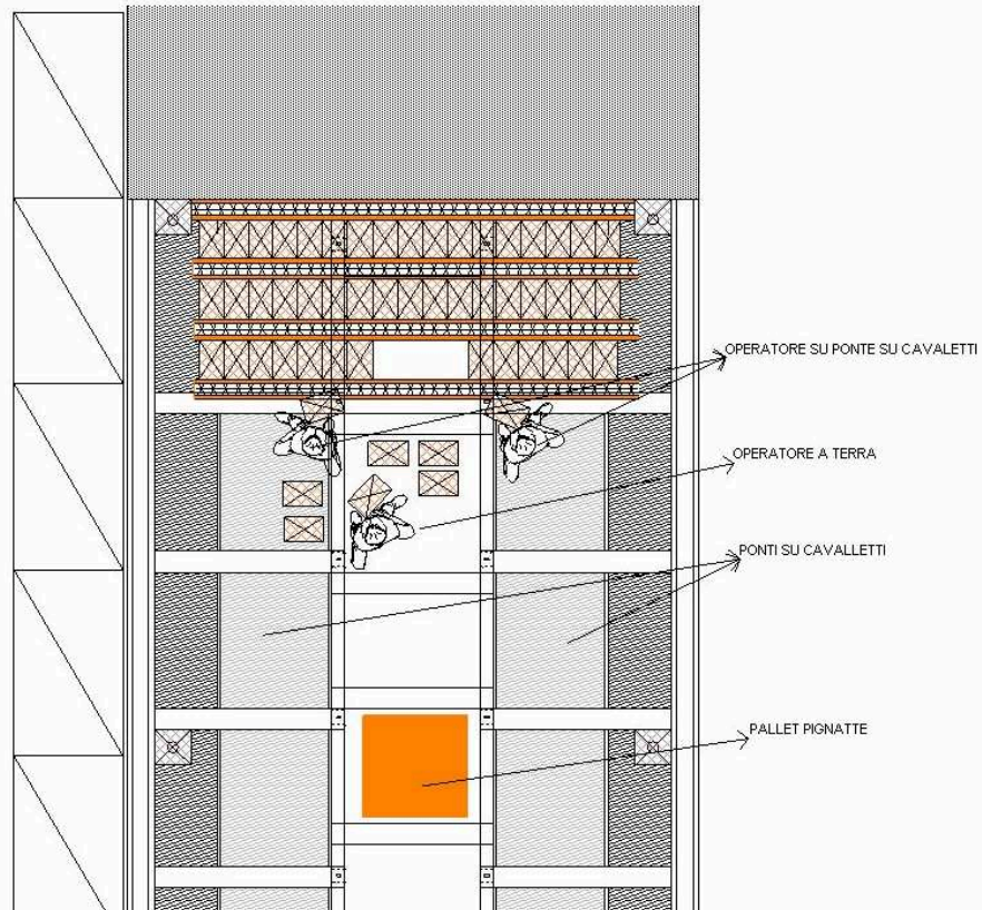
fig. 41 - posa travetti e pignatte dal piano sottostante il solaio – vista planimetrica
