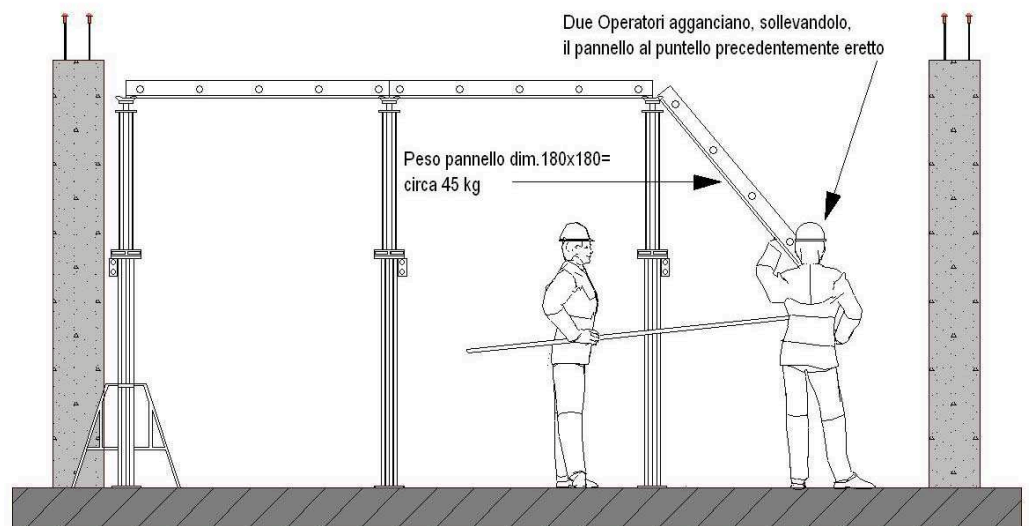
fig. 58 e 59 – posa puntelli e pannelli direttamente agganciati nella testata del puntello
