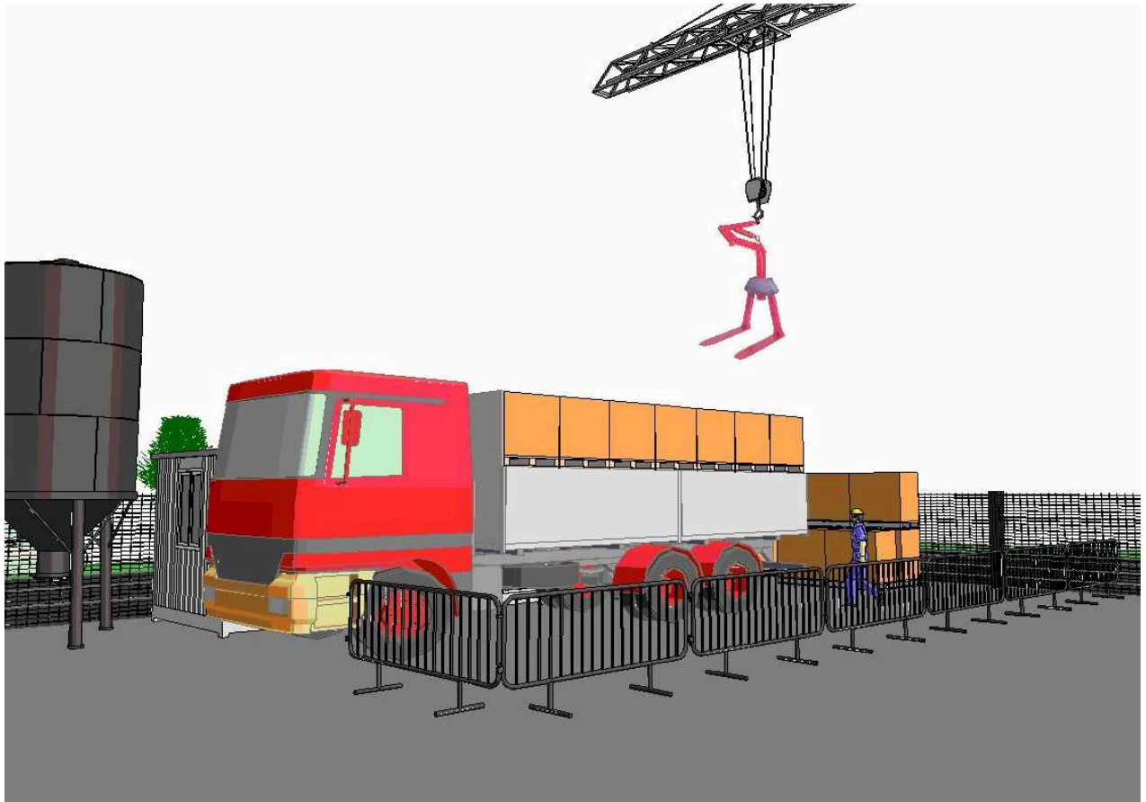
fig. 20 - Scarico laterizi dal camion con uso di gru e forca da cantiere – delimitare l'area di lavoro con transenne metalliche o cavalletti e nastro bianco rosso
