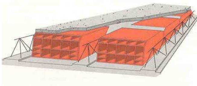
fig. 3 – solai a lastre prefabbricate in c.a con tralicci e blocchi di alleggerimento in laterizio - disegni tratto dal volume Andil "I solai in laterizio"
