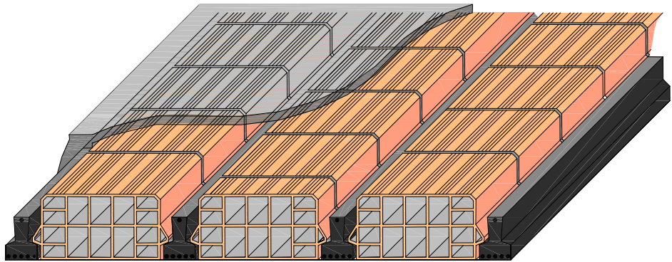
fig. 3 - solaio con travetti in cls armato precompresso
