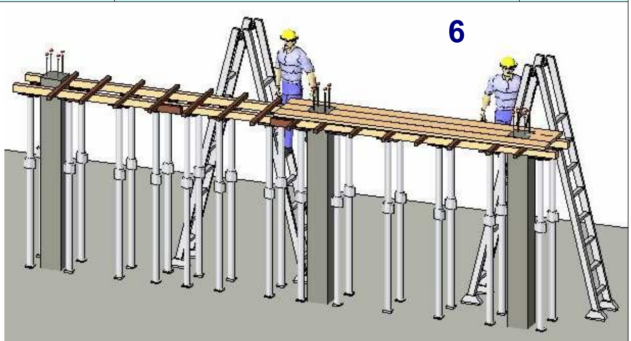
fig. 26 – posa in opera intavolato del banchinaggio trave
