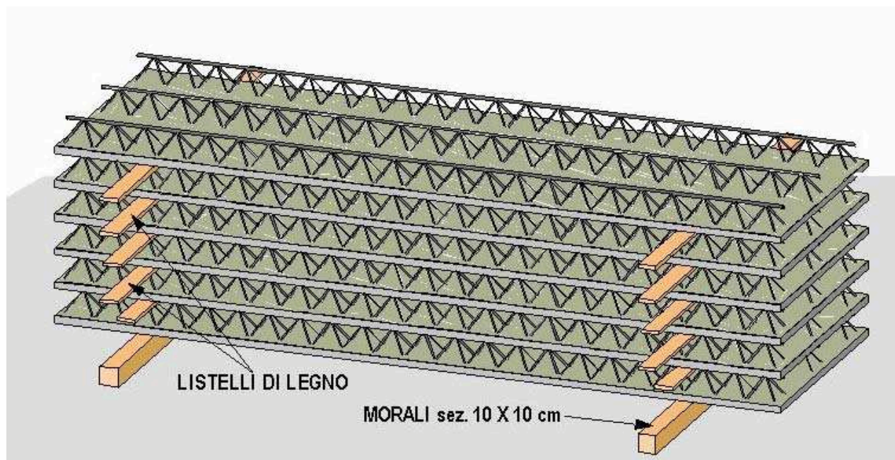
fig.7 – lastre accatastate come previsto dal produttore con interposti listelli di legno o altri materiali REALIZZARE APPOGGI SU PIANI ORIZZONTALI – INTERPORRE LISTELLI SULLA STESSA VERTICALE DEI MORALI
