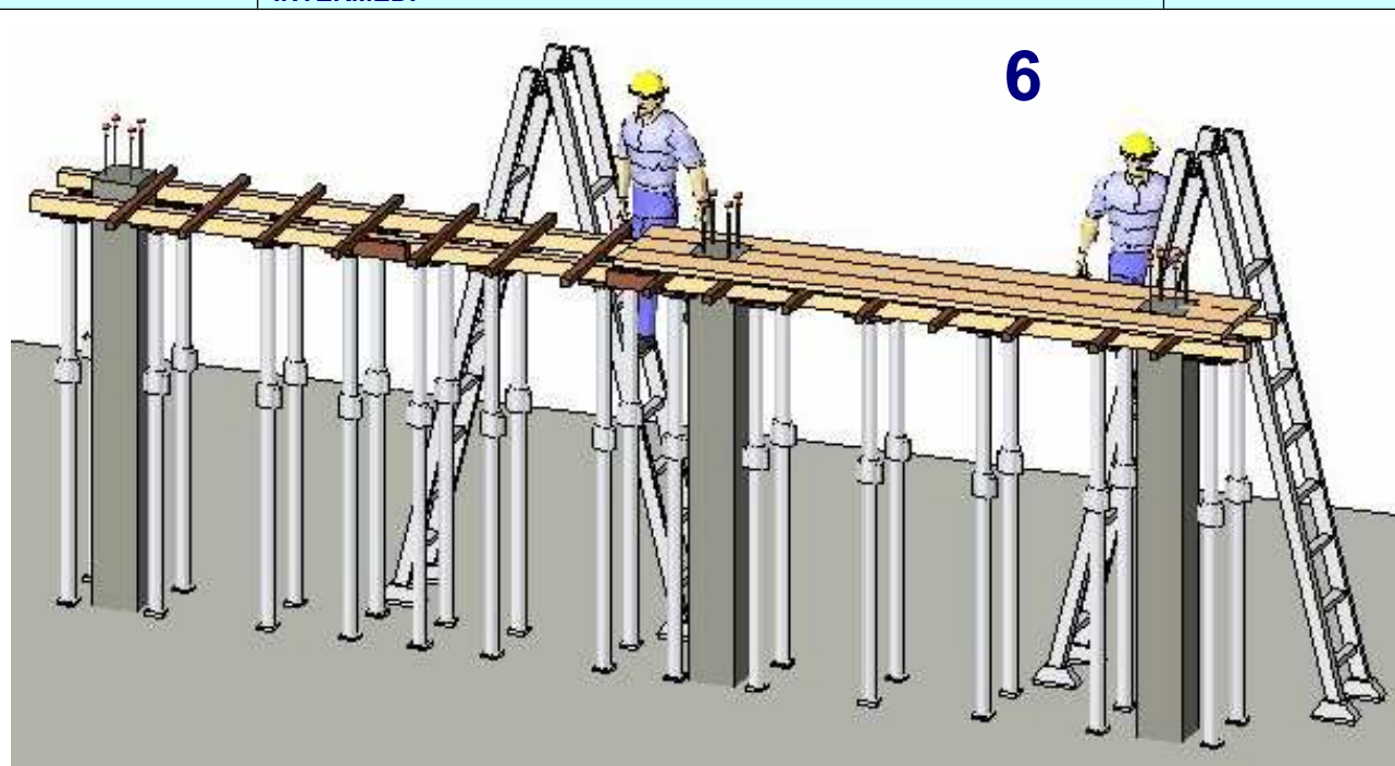
fig. 18 – posa in opera intavolato del banchinaggio trave
