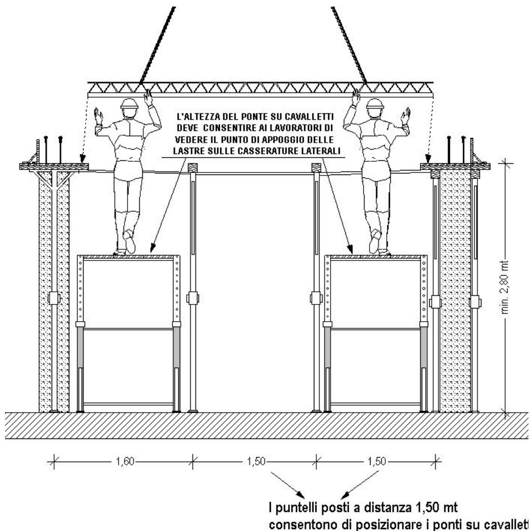
fig. 25 – posa prima lastra dal basso con l'ausilio di ponte su cavalletti
