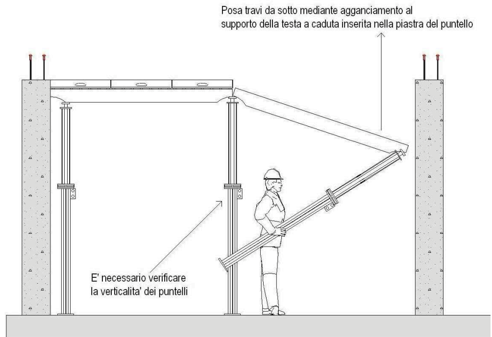
fig. 55 – posa puntelli e travetti dal basso
