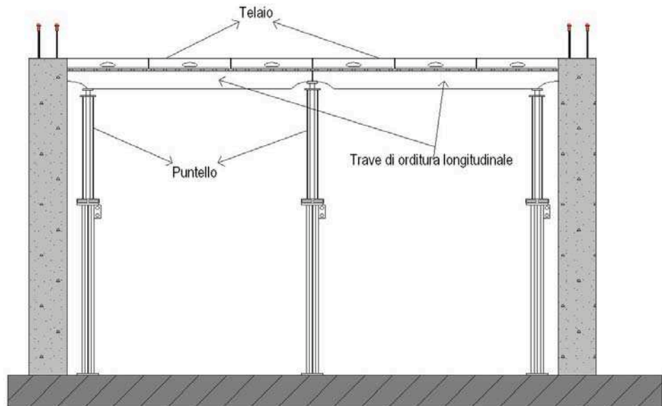
fig. 54 – sistema cassero tipo Peri
