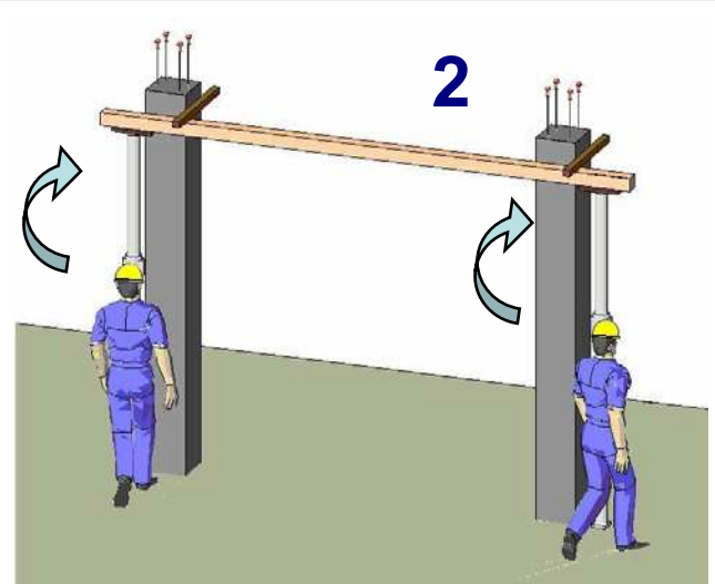
fig. 14 - innalzamento puntello e corrente a livello quotato per il banchinaggio
