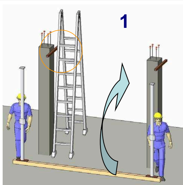
fig. 13 - posa in opera listelli di riferimento chiodati al pilastro e allestimento cavalle a terra con chiodatura puntelli al corrente di sostegno
