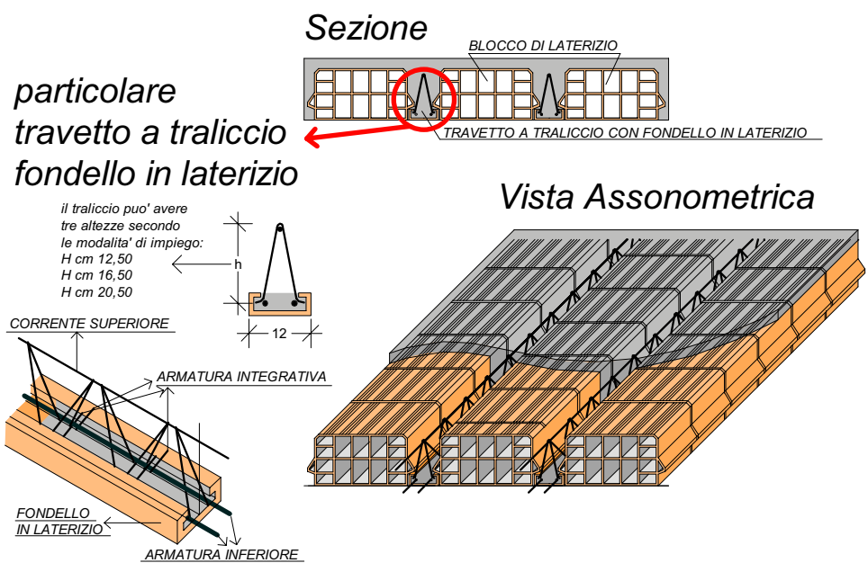
fig. 1 – travetti a traliccio con fondello in laterizio
