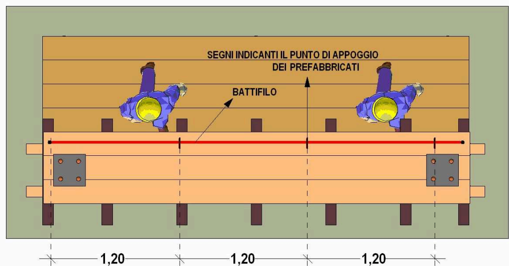
Fig. 33 – segnatura dell'allineamento delle lastre con battifilo e dei punti di giunzione tra una lastra e quella successiva con metro e matita
