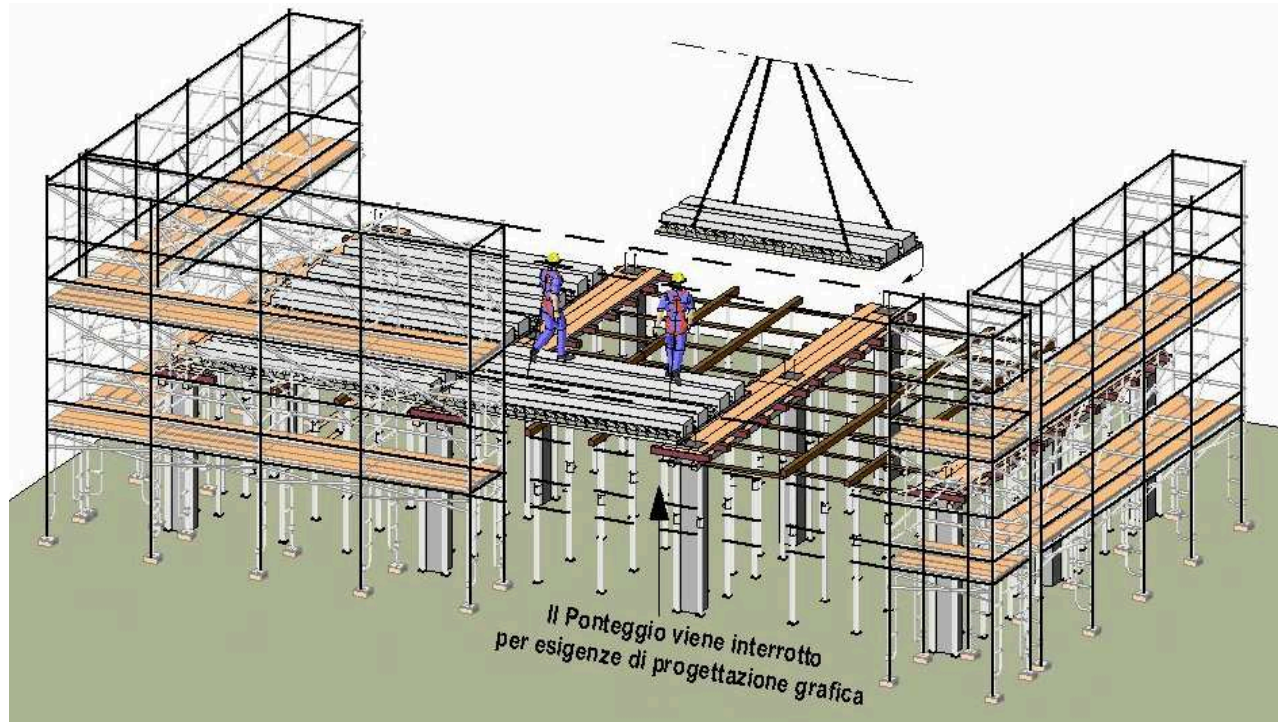
fig. 22 - posa lastre con lavoratori in quota ancorati al traliccio delle lastre già posate
