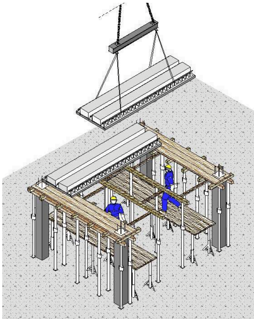
fig.34 – posa lastre dal basso – la movimentazione delle lastre non deve sovrastare l'area di lavoro degli operai
