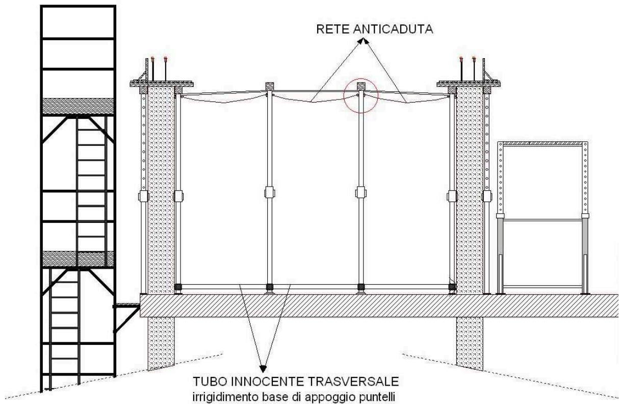
fig. 48 – Uso reti di sicurezza
