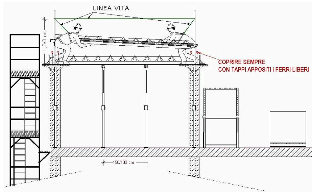
fig. 34 – posa travetti con uso linea vita
