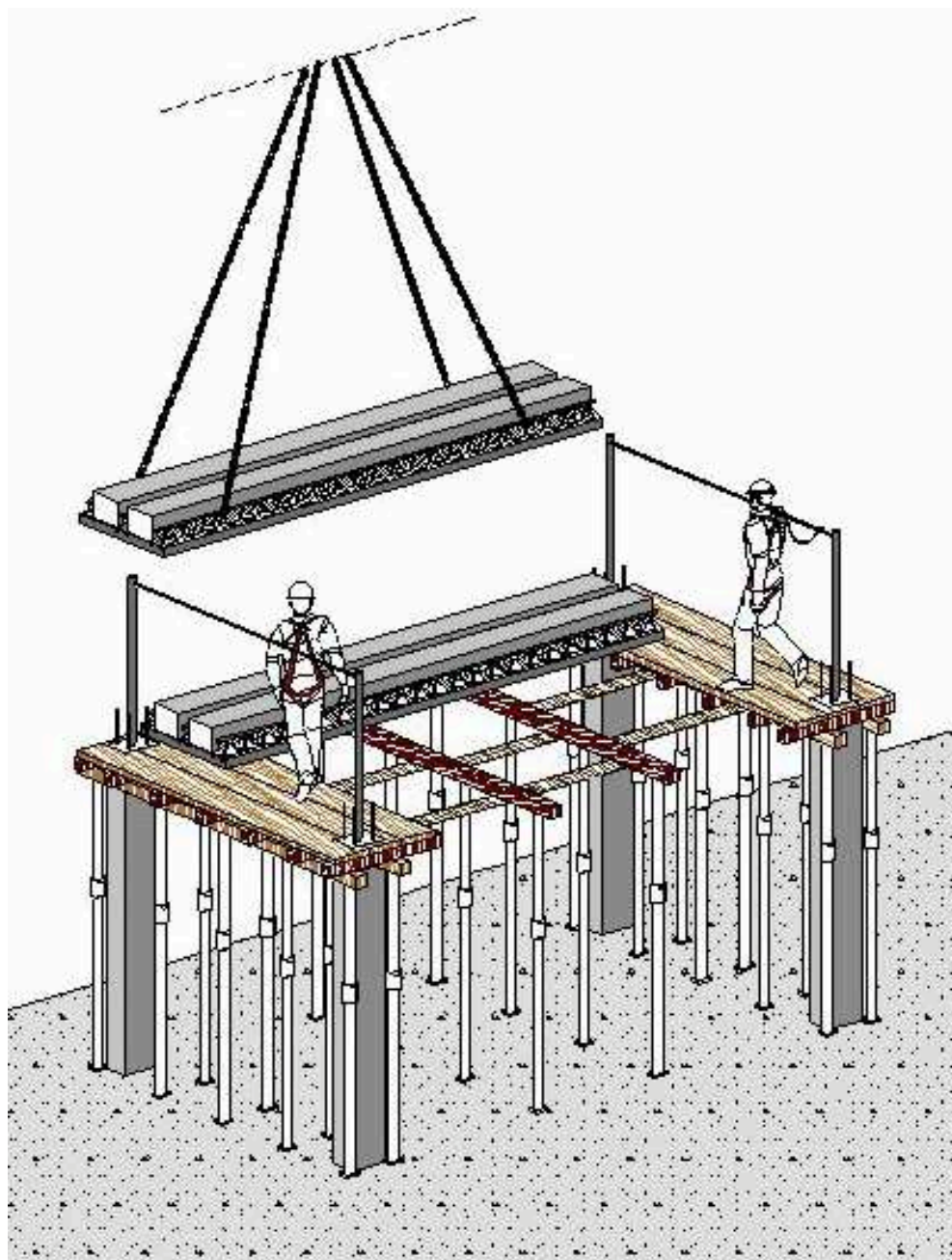
fig. 27 - Posa in opera lastre con ausilio linea vita
