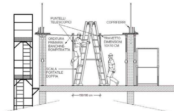
fig. 21 – posa dei puntelli e rompitratta intermedi
