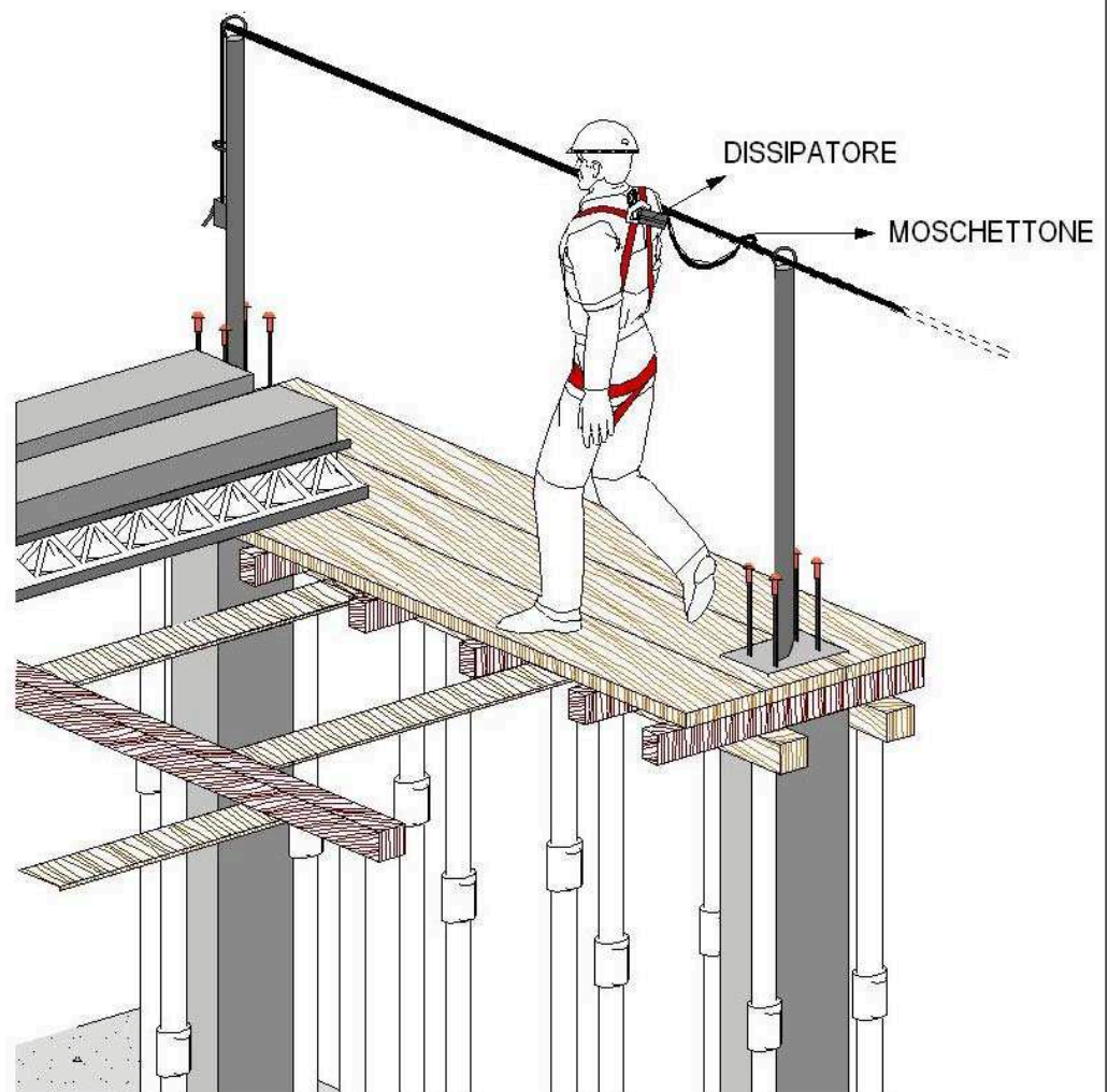
fig. 28 – dettaglio linea vita
