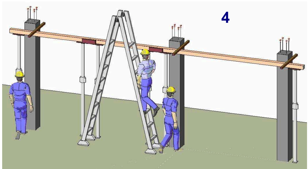
fig. 24 – collegamento - controvento correnti attigue con scala portatile
