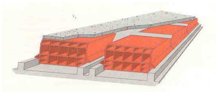
fig. 4 – solai a lastre prefabbricate in c.a con nervature e blocchi di alleggerimento in laterizio - disegni tratto dal volume Andil "I solai in laterizio"
