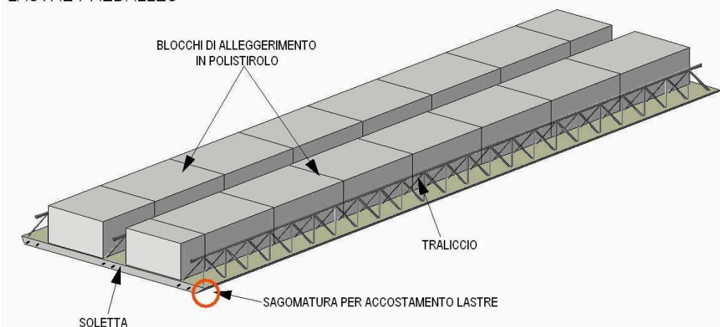
fig. 2 – lastra prefabbricate in c.a con tralicci e blocchi di alleggerimento incorporati in polistirolo
