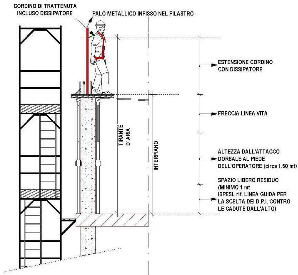
fig. 33 – Posa lastre con uso linea vita tesata tra i montanti annegati nel getto dei pilastri – verifica tirante d’aria
