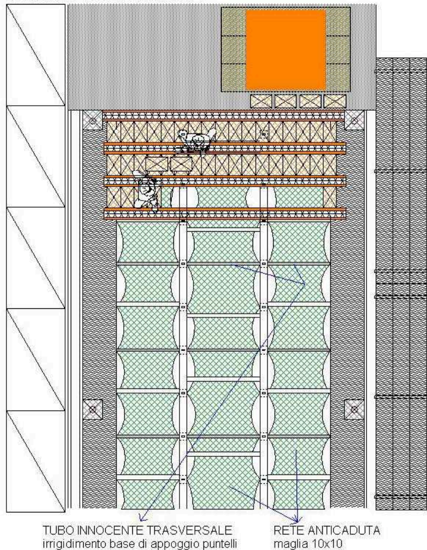
fig. 50 – Uso reti di sicurezza – vista planimetrica
