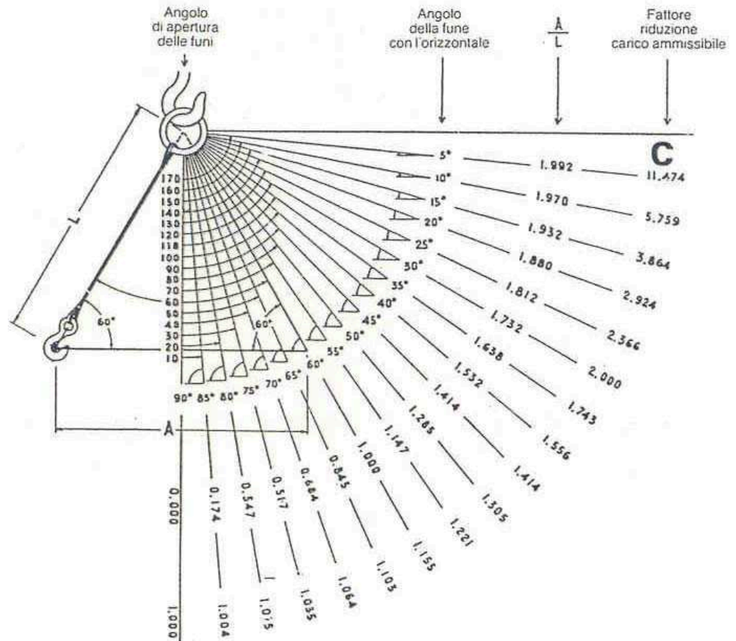
fig. 11 – Fattore di riduzione del carico ammissibile in relazione all'angolo al vertice di due funi o al rapporto A/L , ( A = distanza punti di sollevamento; L = lunghezza catene o fune)
