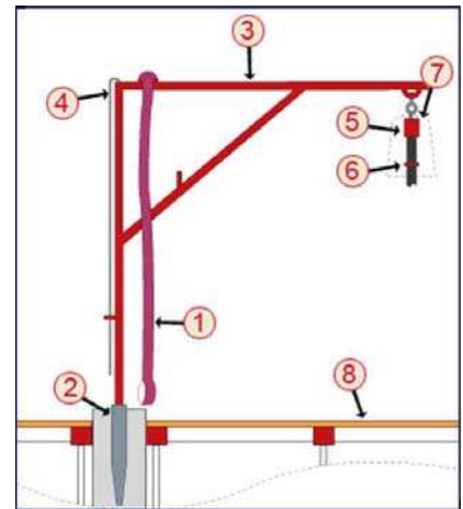
fig. 61 – Esempificazione sistema Alsina per posa dall'alto intavolato continuo
