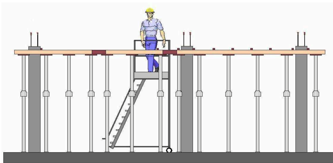
fig. 19 - posa in opera banchinaggio con uso scala a castello di dimensioni idonee alla lavorazione
