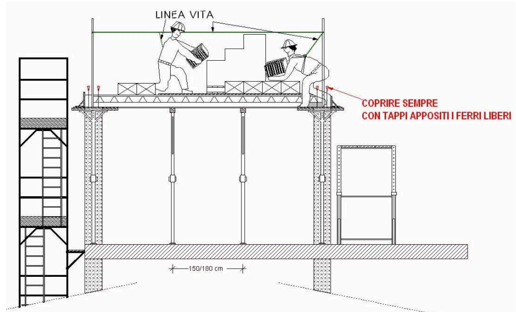
fig. 35 – posa pignatte con ancoraggio linea vita intermedia
