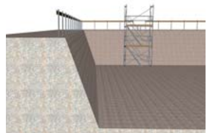
3 Scavo: parapetto singolo sul bordo della scarpata, accesso tramite torre-scala o scala a gradini da cantiere.
