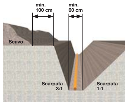
2 Scavo con scarpata 3:1 (sinistra) e 1:1 (destra)
