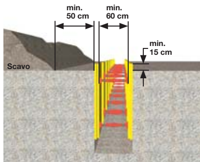
1 Scavo con sbadacchio
